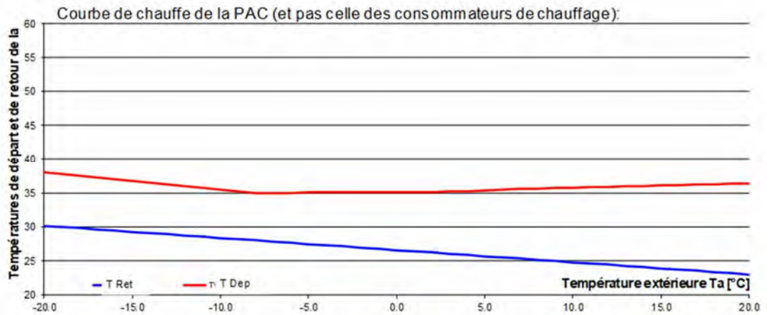
Fig. 5-2 Températures de départ et de retour dans PACesti
